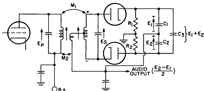
Fig. 33—Ratio-detector circuit.
